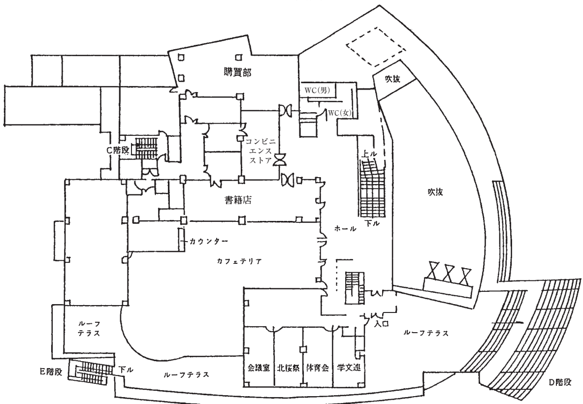
2階平面図
