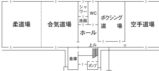
1 階 平 面 図
