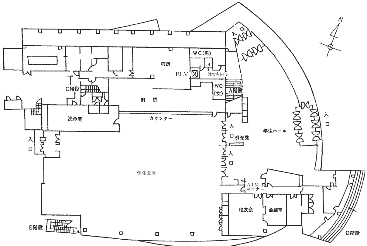
1階平面図
